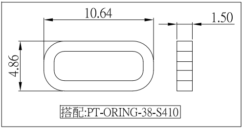
加防水圈示意图
